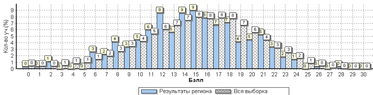
Распределение первичных баллов участников НИКО в 6 классах
