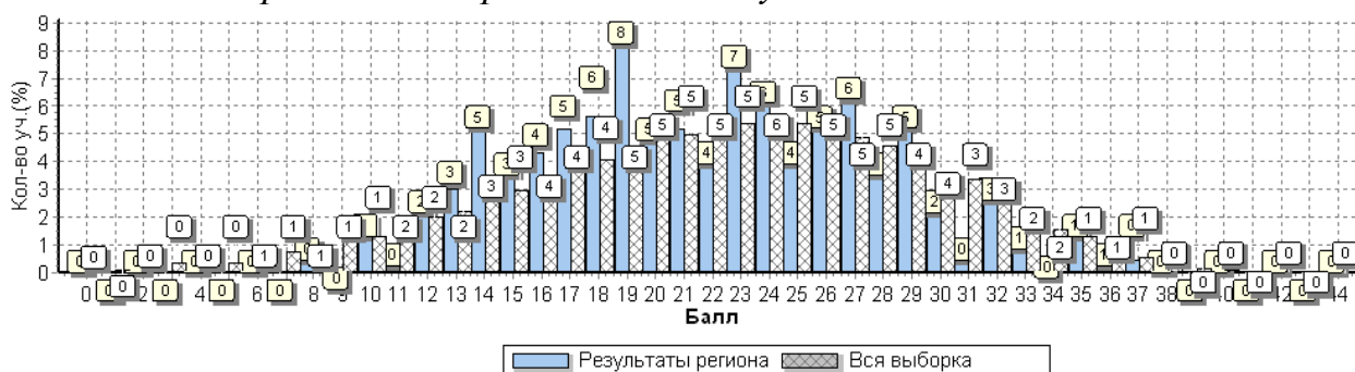
Распределение первичных баллов участников НИКО в 8 классах
